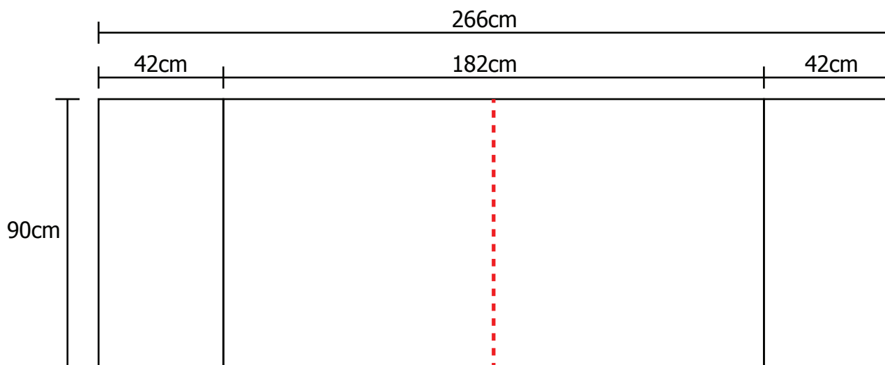
גוף הדלפק
